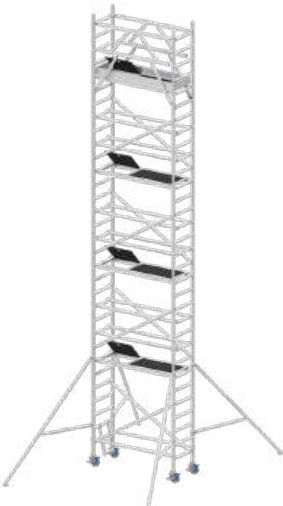
RS075x185x800
