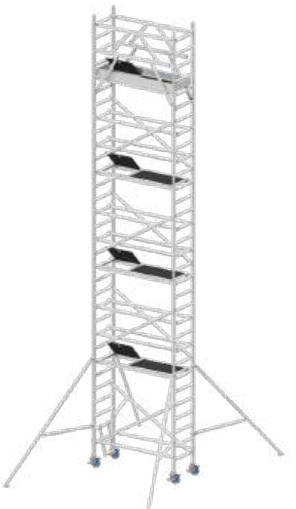
RS075x185x800
