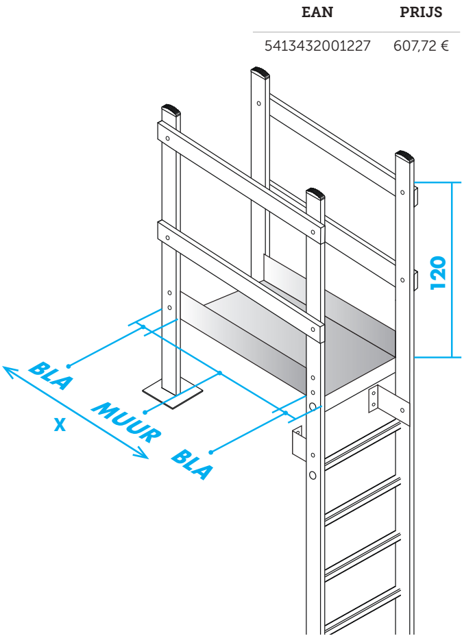
Overstapplatform in traanplaat "bruut" X = 2 x BLA + MUURDIKTE
