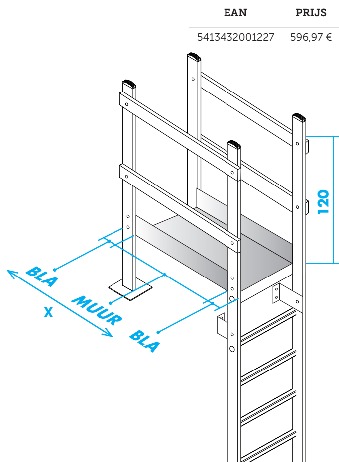
Overstapplatform in traanplaat "bruut" X = 2 \times \text{BLA} + \text{MUURDIKTE}
